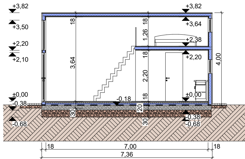
A-A METSZET
