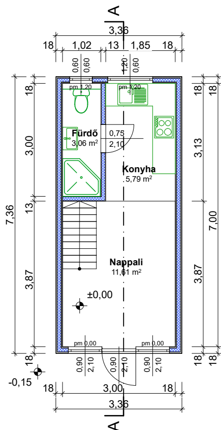
FÖLDSZINT ALAPRAJZ
