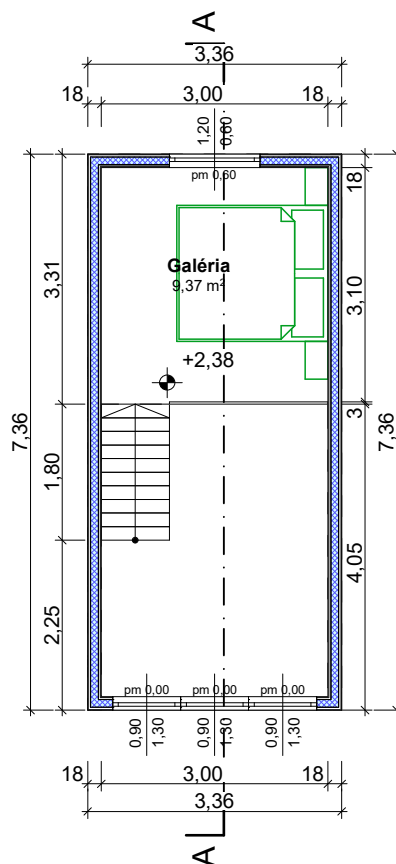
GALÉRIA ALAPRAJZ
